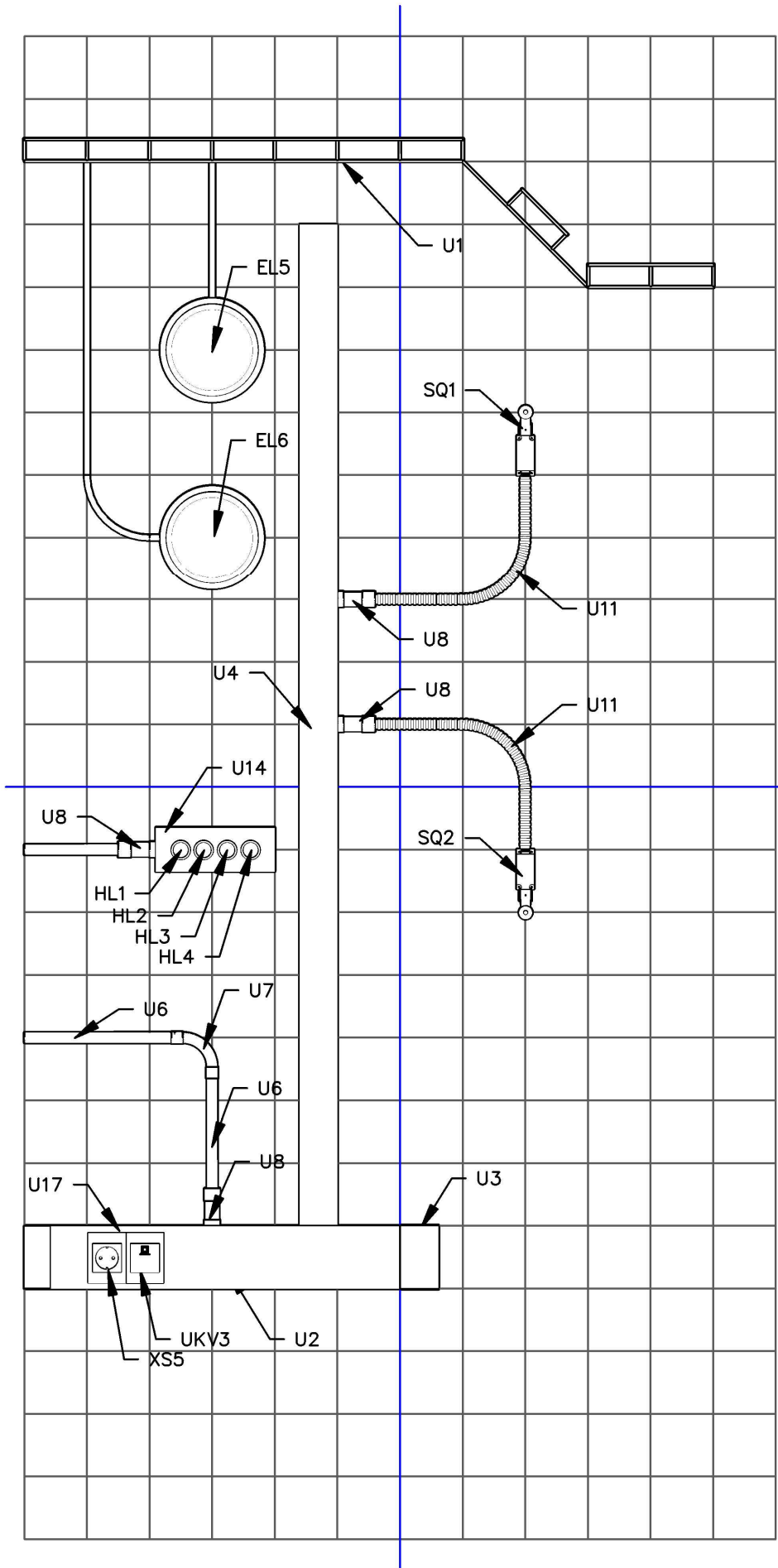
Монтажная схема вид "В"
